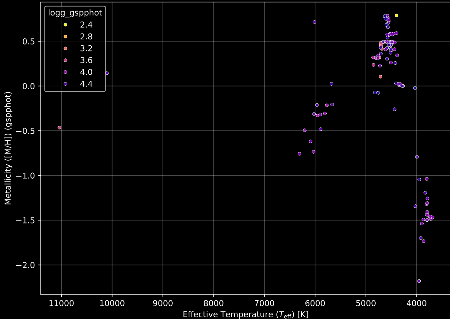
APOGEE DR17 Field: [FORNAX] Stellar Population Parameters (n= 127)
